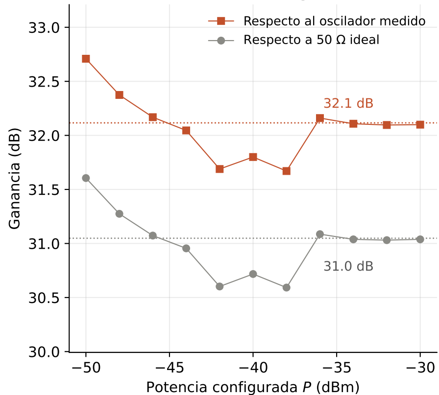
(b) Ganancia del amplificador
