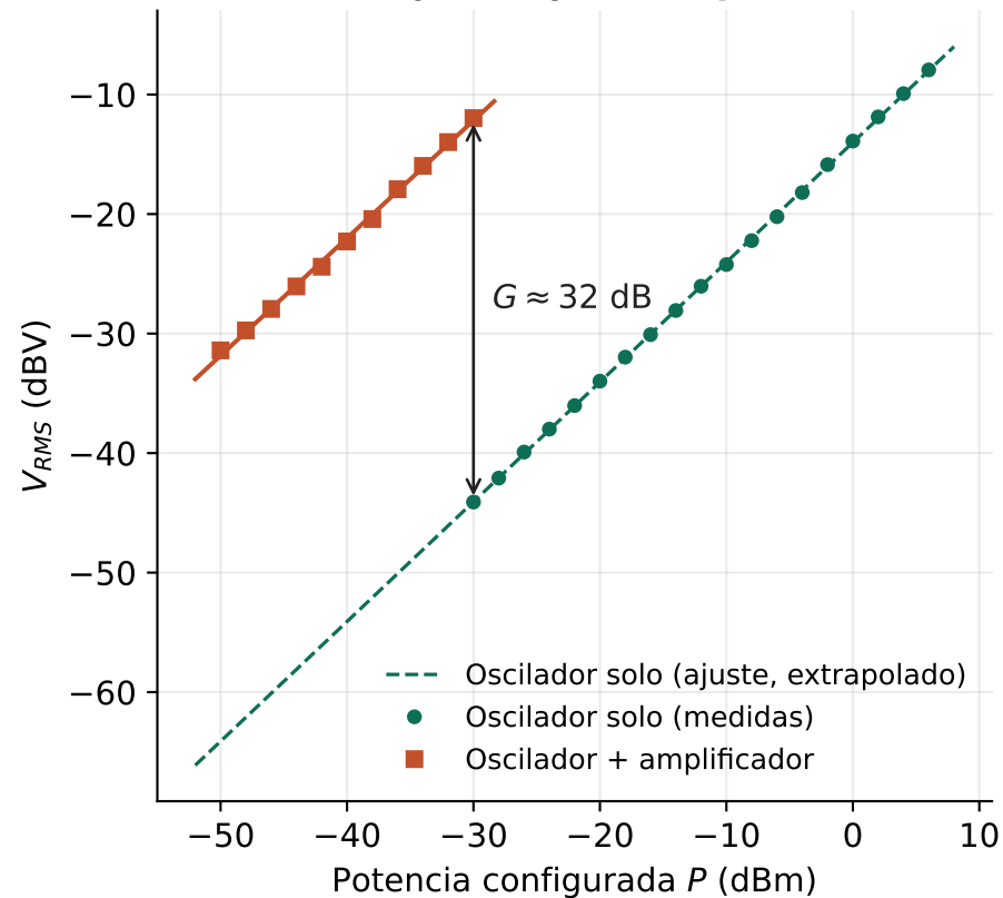
(a) Voltaje con y sin amplificador
